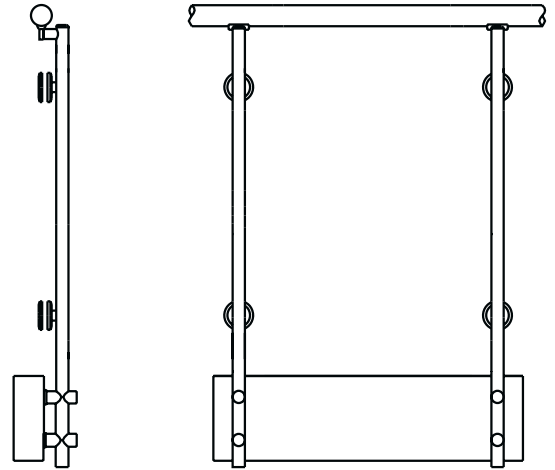
Cam Tutuculu Düz Merdiven Kúpeřtesi 8502.22 D
