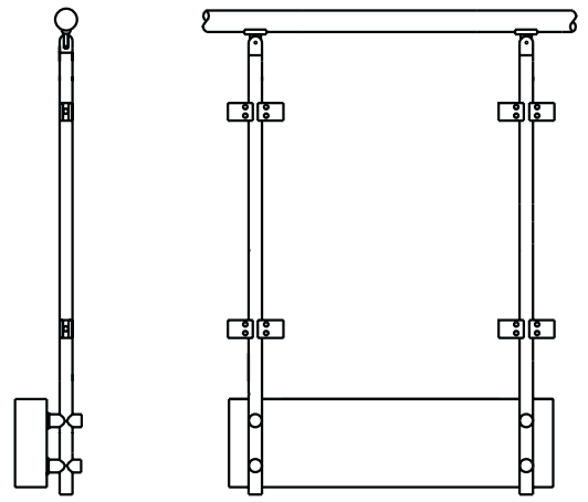
Cam Tutuculu Düz Merdiven Kúpeřtesi 8501.12 D
