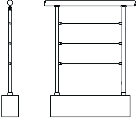
Üç Paralelli Halat Gergili Düz Merdiven Küpeştesi
