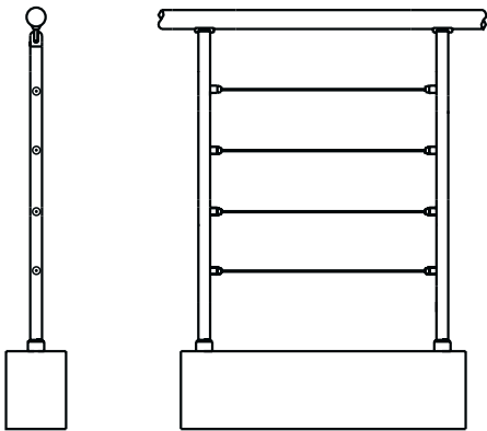
Dört Paralelli Halat Gergili Düz Merdiven Küpeştesi
