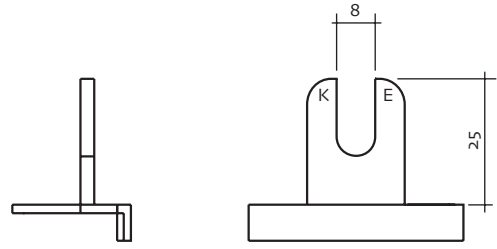
Kısa Dil
