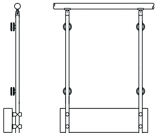
Cam Tutuculu Düz Merdiven Kúpeřtesi 8502.21 D
