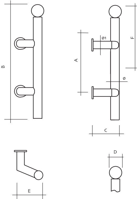
Kaynaklı Ayak
