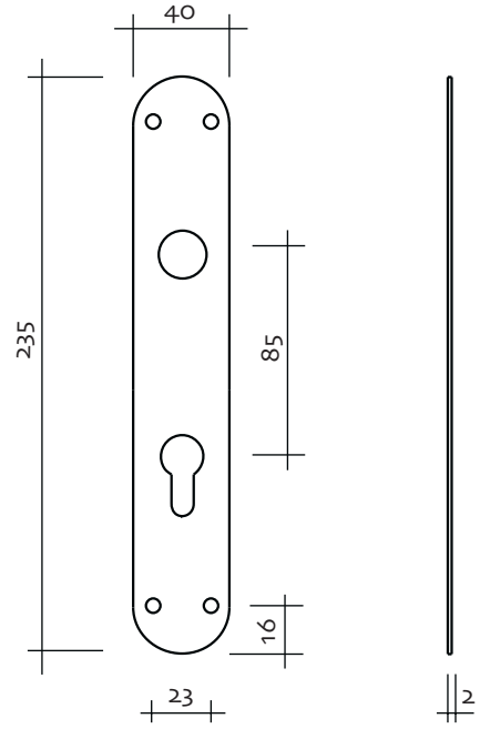
3100.02 Paslanmaz Çelik
