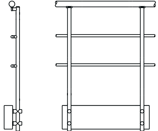
 ki Paralelli D z Merdiven K peřtesi 8302.22 D
