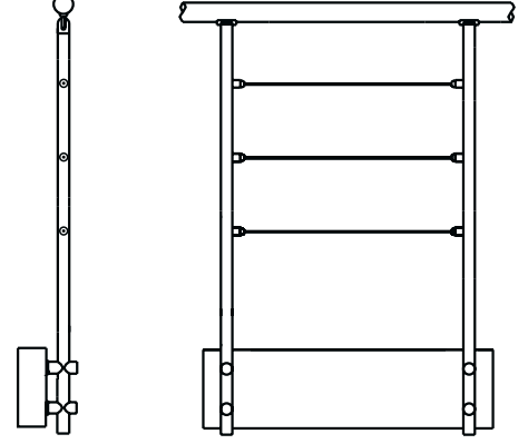
Üç Paralelli Halat Gergili Düz Merdiven Küpeştesi
