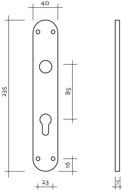
3100.00 Alüminyum
