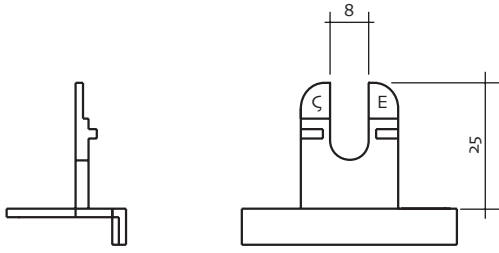
Çift Eksenli Dil
