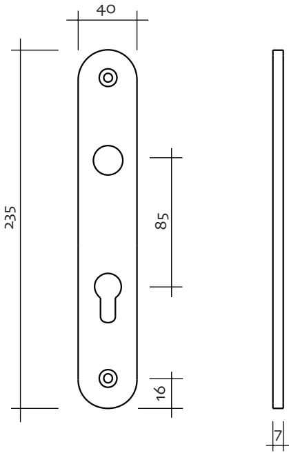
3100.03 Paslanmaz Çelik
