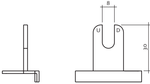
Uzun Dil
